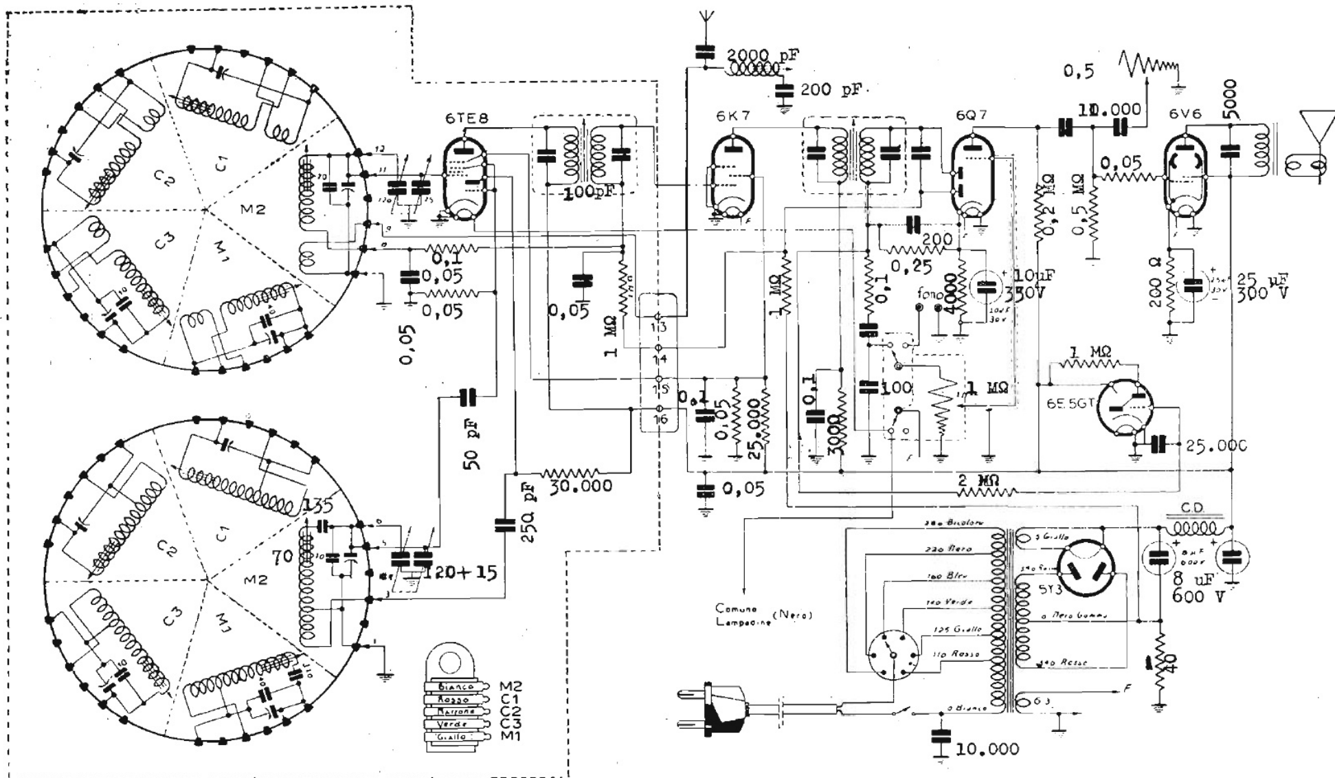
PEBA RADIO - Mod. A/505, con variatore di gamma a tamburo rotante. Onde medie 1 da 320 a 580 m; onde medie 2 da 195 a 320 m; onde corte da 34 a 54 m, da 21 a 34 m e da 12,5 a 21 m: MF a 467 kc/s.
